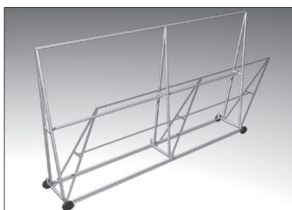
Тележка для хранения и транспортировки полотна сдвижных ворот.
