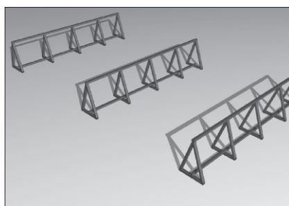
Стапели для сборки полотна ворот. Верхние балки покрыть мягким материалом (ковролин, линолеумом и т.п.) Материал — труба 60х30 мм.
